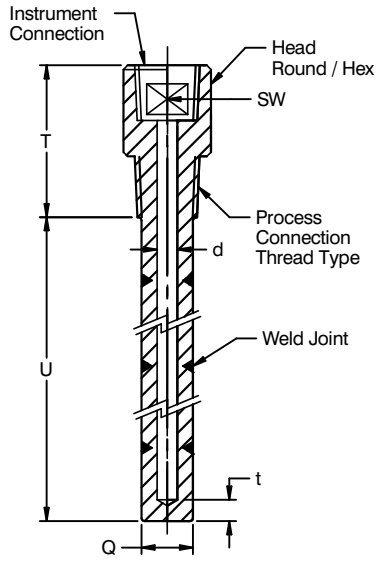
Straight Thermowell
