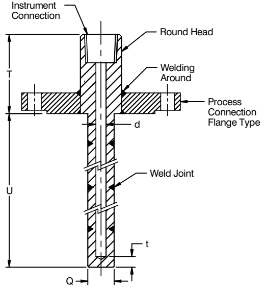
Straight Thermowell
