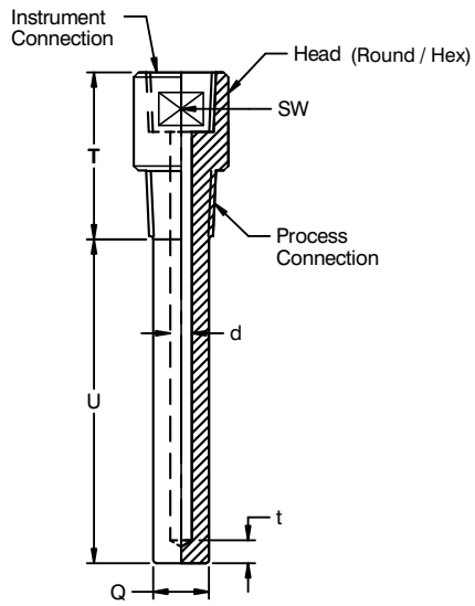
Straight Thermowell
