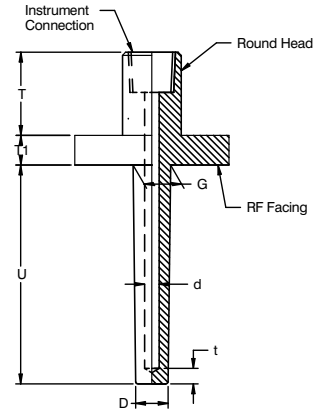
Taper Thermowell
