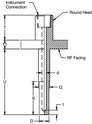
Step Thermowell
