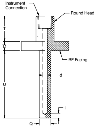
Straight Thermowell
