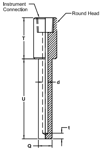
Straight Thermowell
