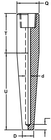
Taper Thermowell
